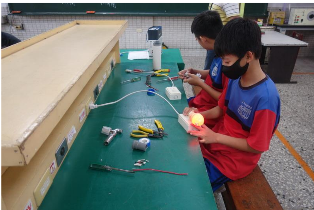
同學製作完成使用小夜燈測試功能情形
